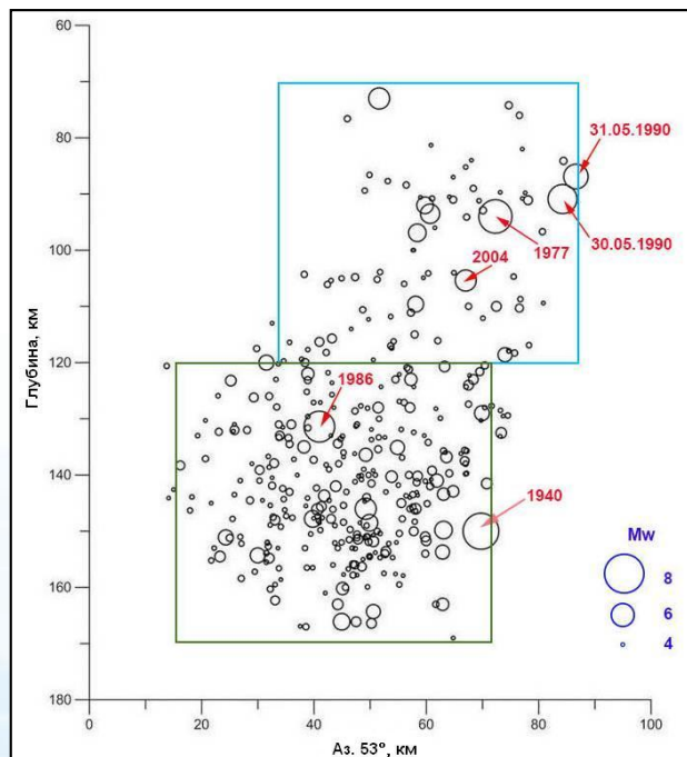
Poziția hipocentrelor de cutremur în regiunea Vrancea
