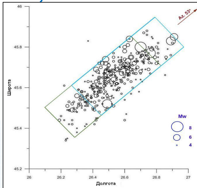
Epicentrele cutremurelor din Vrancea cu M_w \geq 4 pentru perioada 1968-2018
